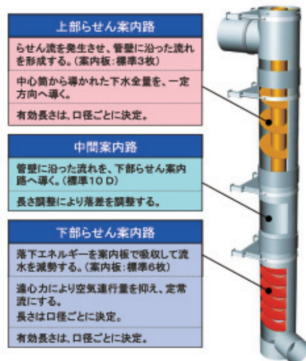
図ー1 ドロップシャフトの標準構造
