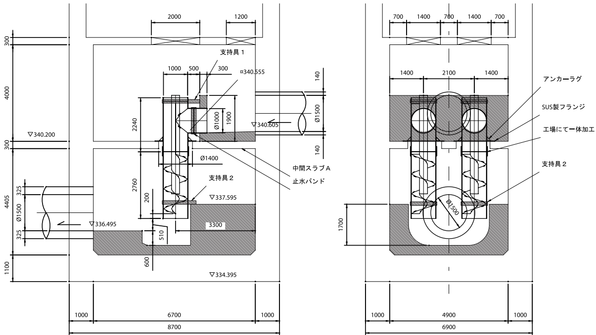
図-2 今回リポートしたドロップシャフトの断面図
