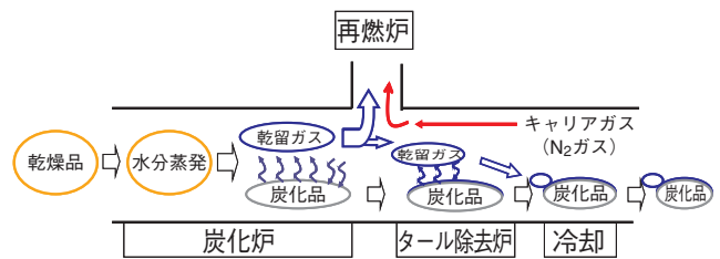
図一7 炉内正圧時の炭化品汚染概念図
