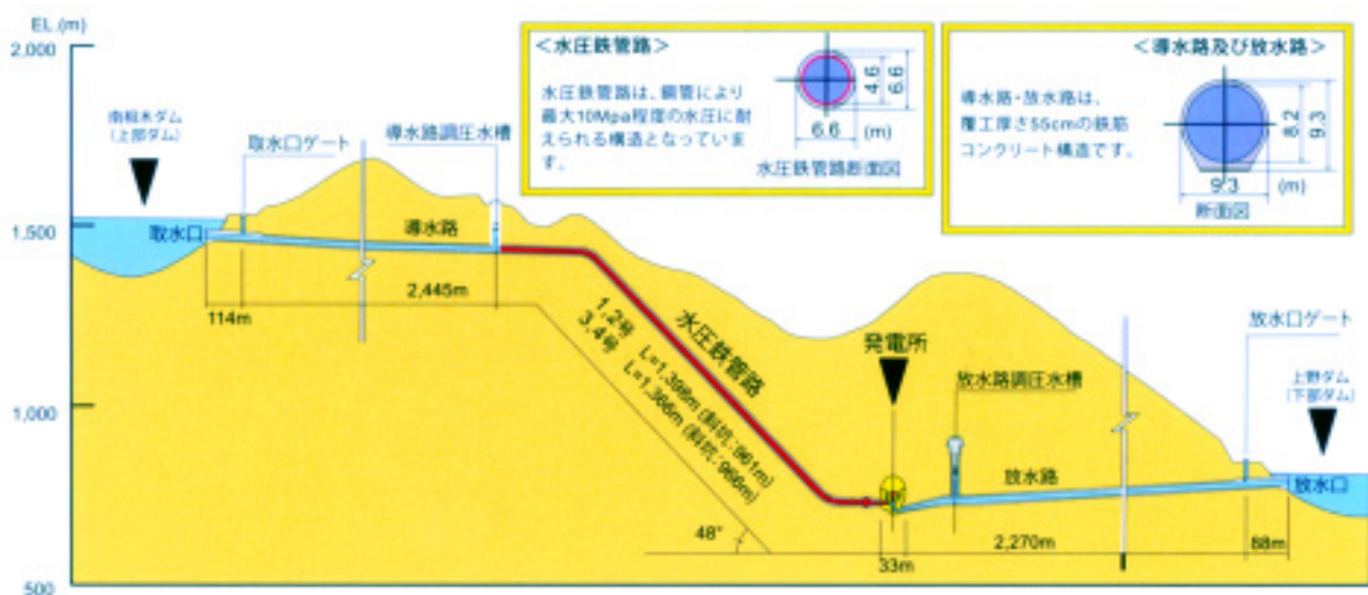
神流川発電所の縦断面図
