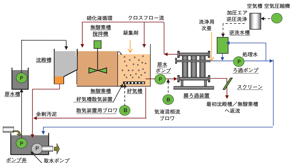
サテライトMBR実証設備のフロー図
