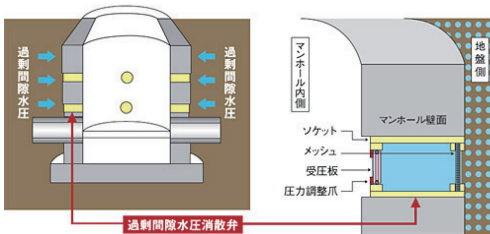
図-2 フロートレス工法概要図
