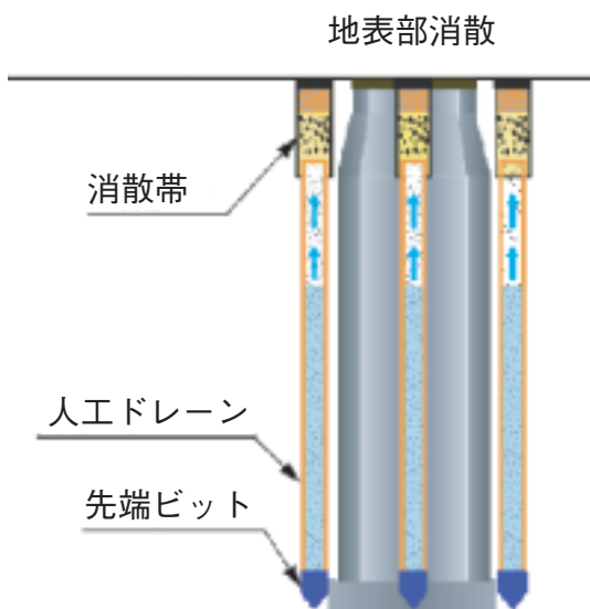
図-3 アースドレーン工法概要図
