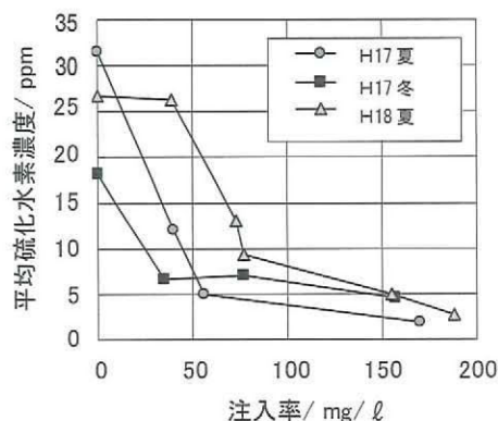
図一六 ポリ鉄注入における抑制効果1 (平均BOD: 280mg/ℓ)
