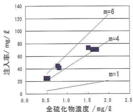
図一八 ポリ鉄の経験的係数の検討
