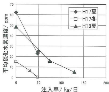
図一5 硝酸塩注入の抑制効果（ L=4\text{ km} ） （経験的係数=0.55， 120\sim 200\text{ kg/day} ）
