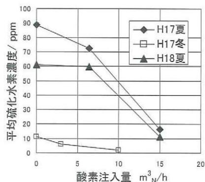
図一3 酸素注入の抑制効果（ L=4\text{ km} ） （経験的係数=1： 3.0, 6.4\text{m}^3/\text{h} ）
