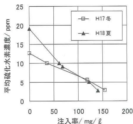
図一七 ポリ鉄注入の抑制効果2 (平均BOD: 180mg/ℓ)
