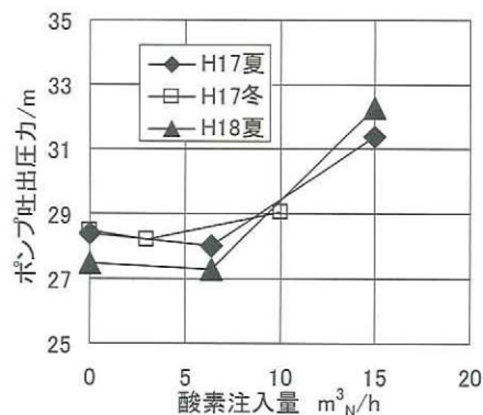
図一4 酸素注入の圧損上昇（ L=4\text{ km} ） （経験的係数=1： 3.0, 6.4\text{m}^3/\text{h} ）
