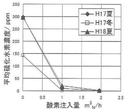
図一2 酸素注入の抑制効果（ L=1\text{ km} ） （経験的係数=1： 1.9\text{m}^3/\text{h} ）
