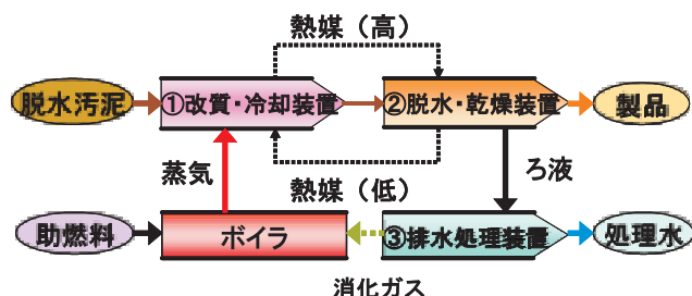
図-1 ブロックフロー
