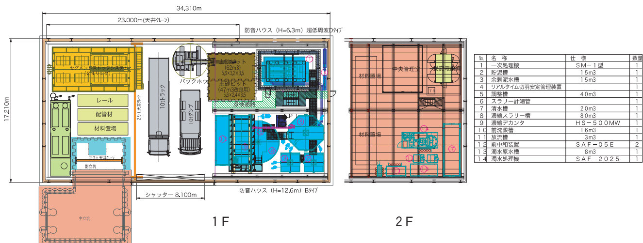
設備配置図
