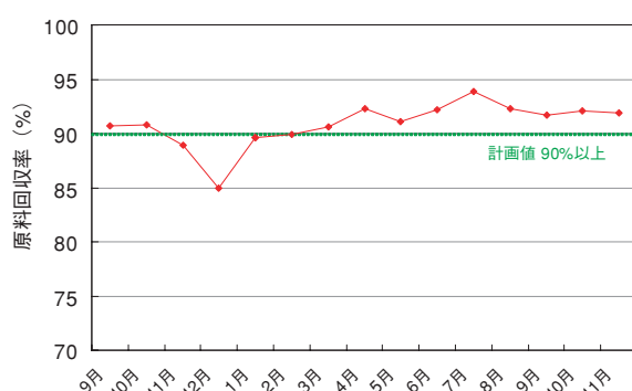
図－4 平均原料回収率の推移
