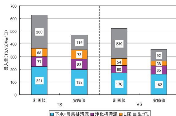
図-3 各バイオマスの受入TS量とVS量
