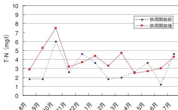
図－９ 放流水のT-N推移
