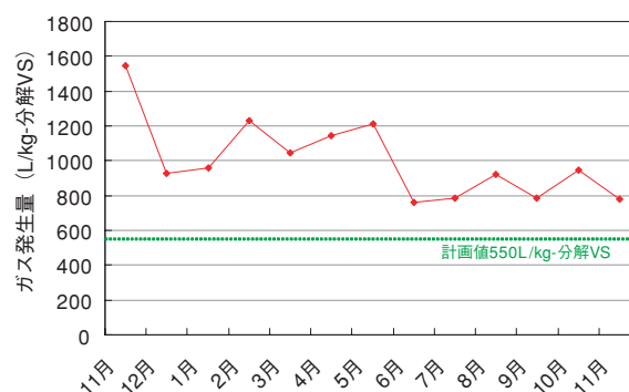
図－6 分解VSあたりガス発生量の推移
