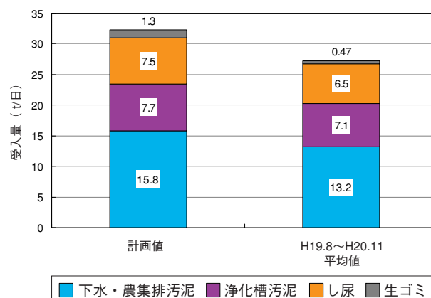
図-2 各バイオマスの受入量
