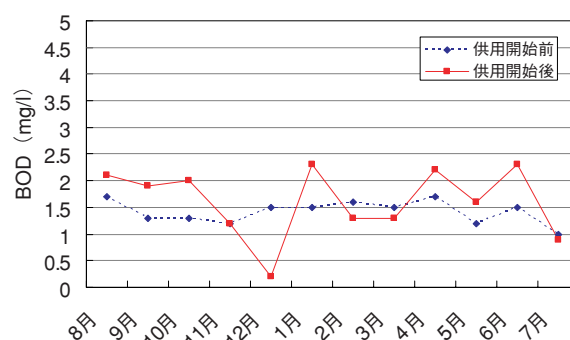
図－８ 放流水のBOD推移
