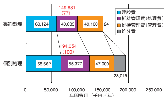
図-10 LCC比較（実績処理量ベース）
