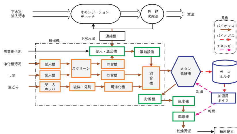
図ー1 処理フロー図
