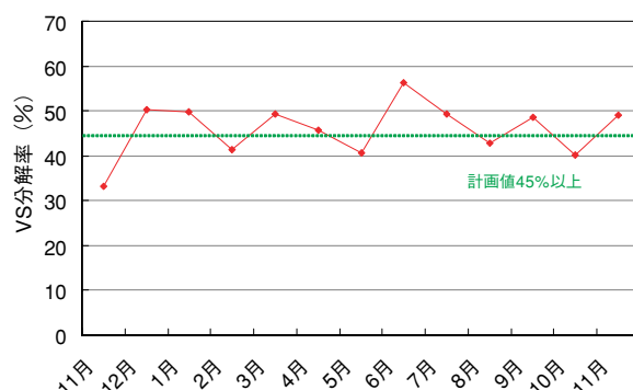
図－5 VS分解率の推移
