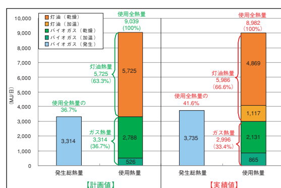
図－7 施設熱利用状況
