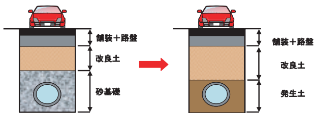
図一 5 発生土の管きょ基礎への利用
