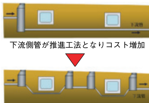
図-3 改良型伏越しの連続的採用
