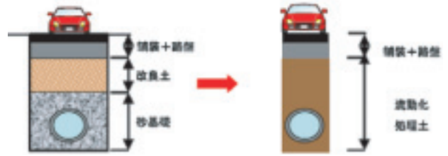
図一 6 流動化処理土の管きょ施工への利用
