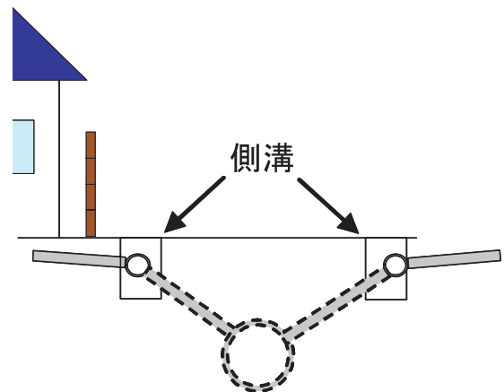
図一 7 側溝を活用した管きょ施工
