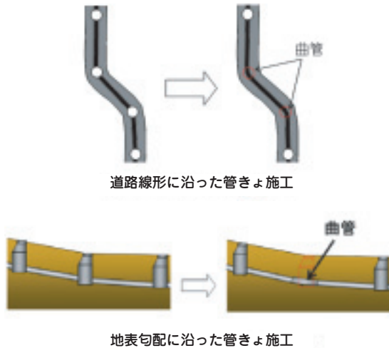
図一 4 道路線形に合わせた施工
