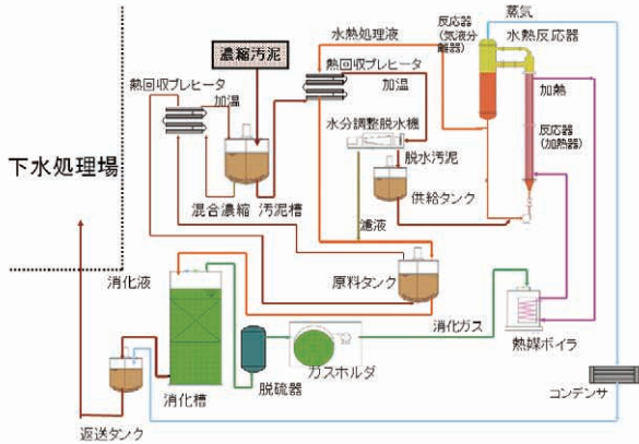
図-5 実証プラントフロー
