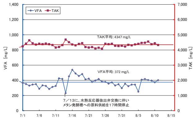
図-8 有機脂肪酸とアルカリ度の推移
