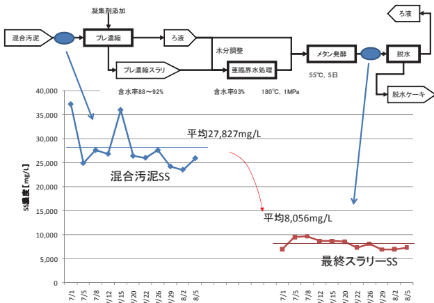
図-6 供給汚泥と最終スラリーのSS濃度変化
