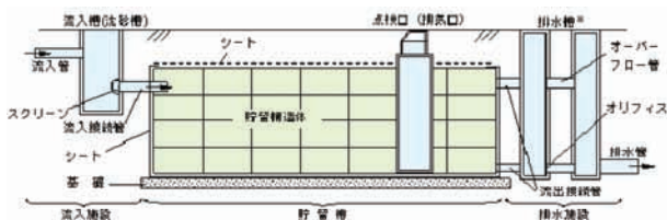
図ー1 プラ貯留施設
