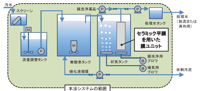
図-1 本法フロー
