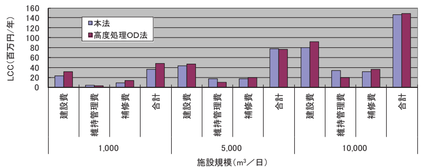
図-6 ライフサイクルコストに関する本法と従来法の比較
