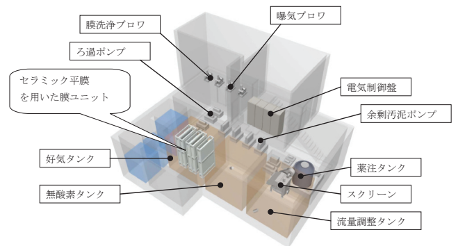
図-2 本法施設の配置イメージ
